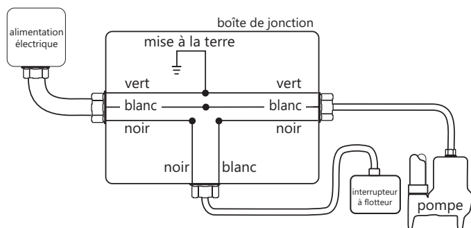
Figure 1. Câblage direct de pompes automatiques monophasées 115 V ou 208/230 V
