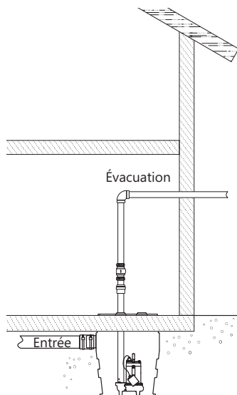
Figure 3. Installation de puisard type (particuliers peuvent varier)
