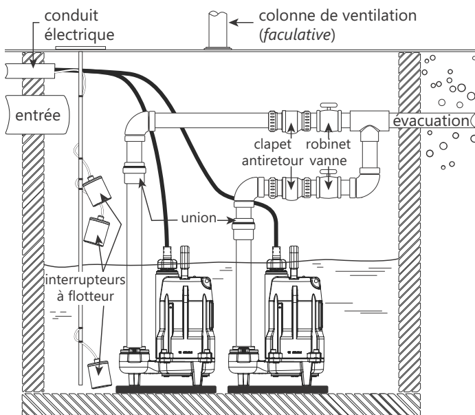
Figure 5. Installation type du système double (particuliers peuvent varier)
