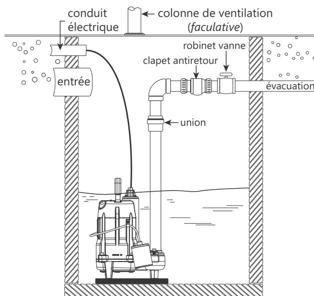
Figure 4. Installation type du système à une pompe (particuliers peuvent varier)
