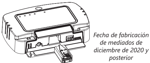
Figura 2. 9V instalación de batería con bandeja
