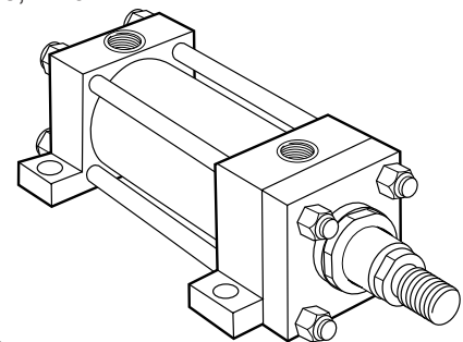
Models 67, 68 ISO Styles ME5, ME6
