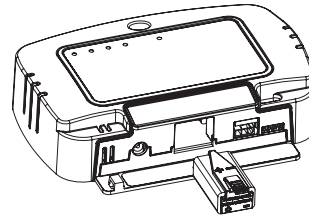
Figure 2. Installation de la batterie 9 V avec plateau
