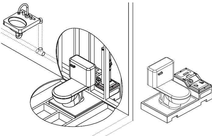
Figure 1. Installation type avec finition et Orientation facultative de la cuvette
