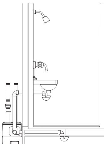
Figure 2. Vue latérale d'une douche surélevée
