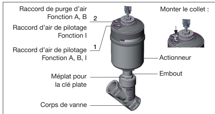
Fig. 3 : Montage
