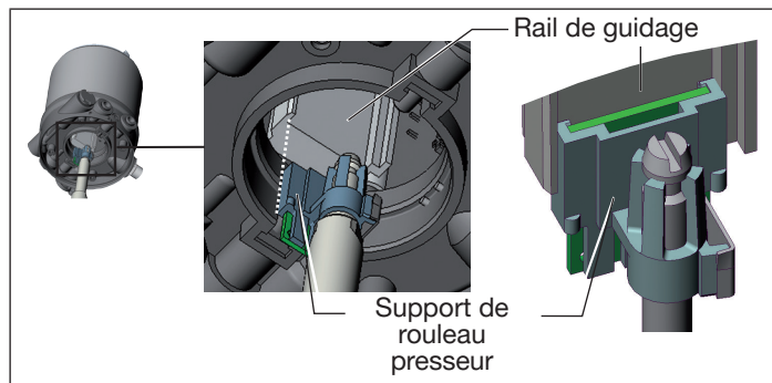
Fig. 5 : Disposition du support de rouleau presseur
